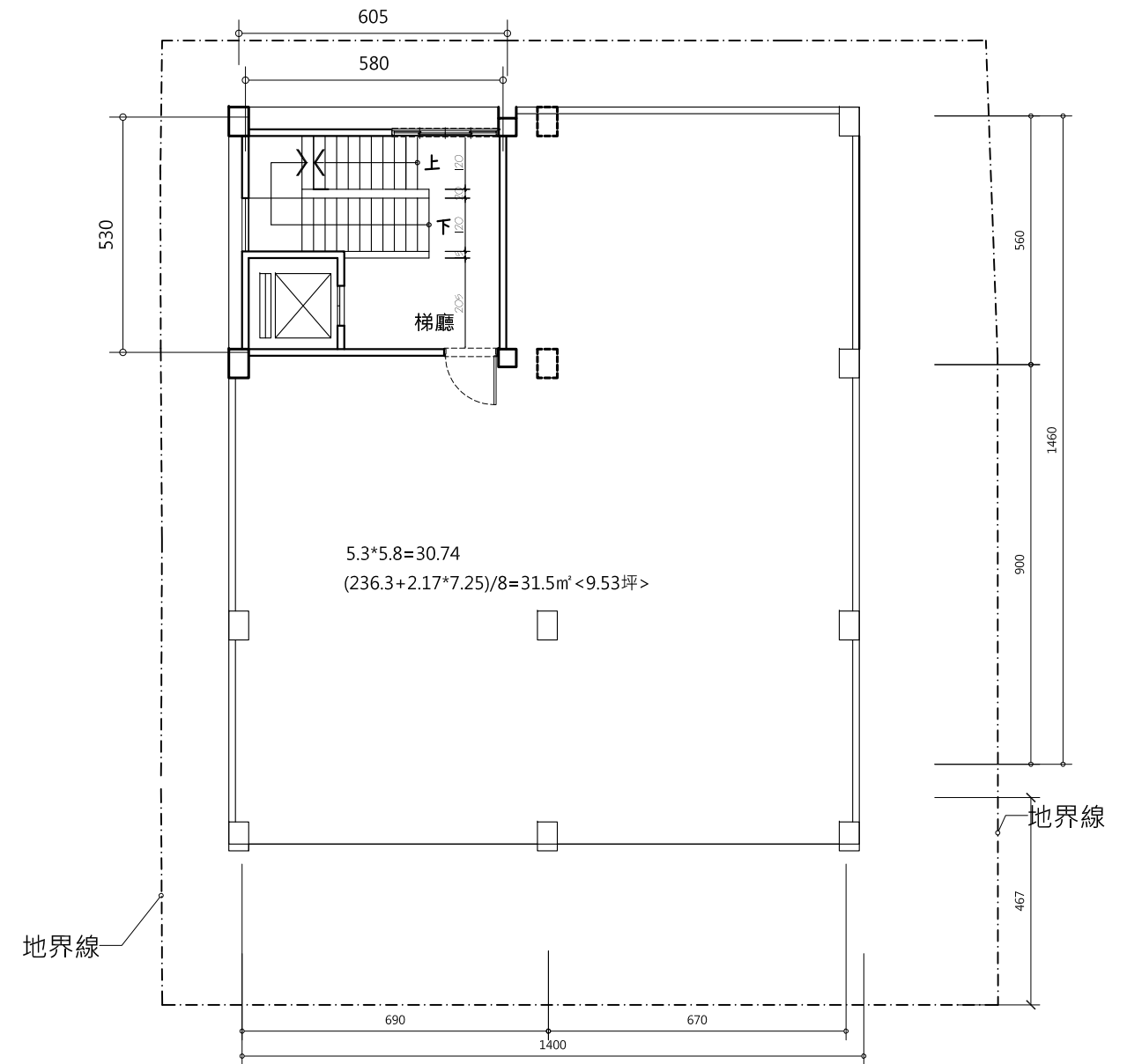
2 屋突一層平面圖 Scale=1/150
